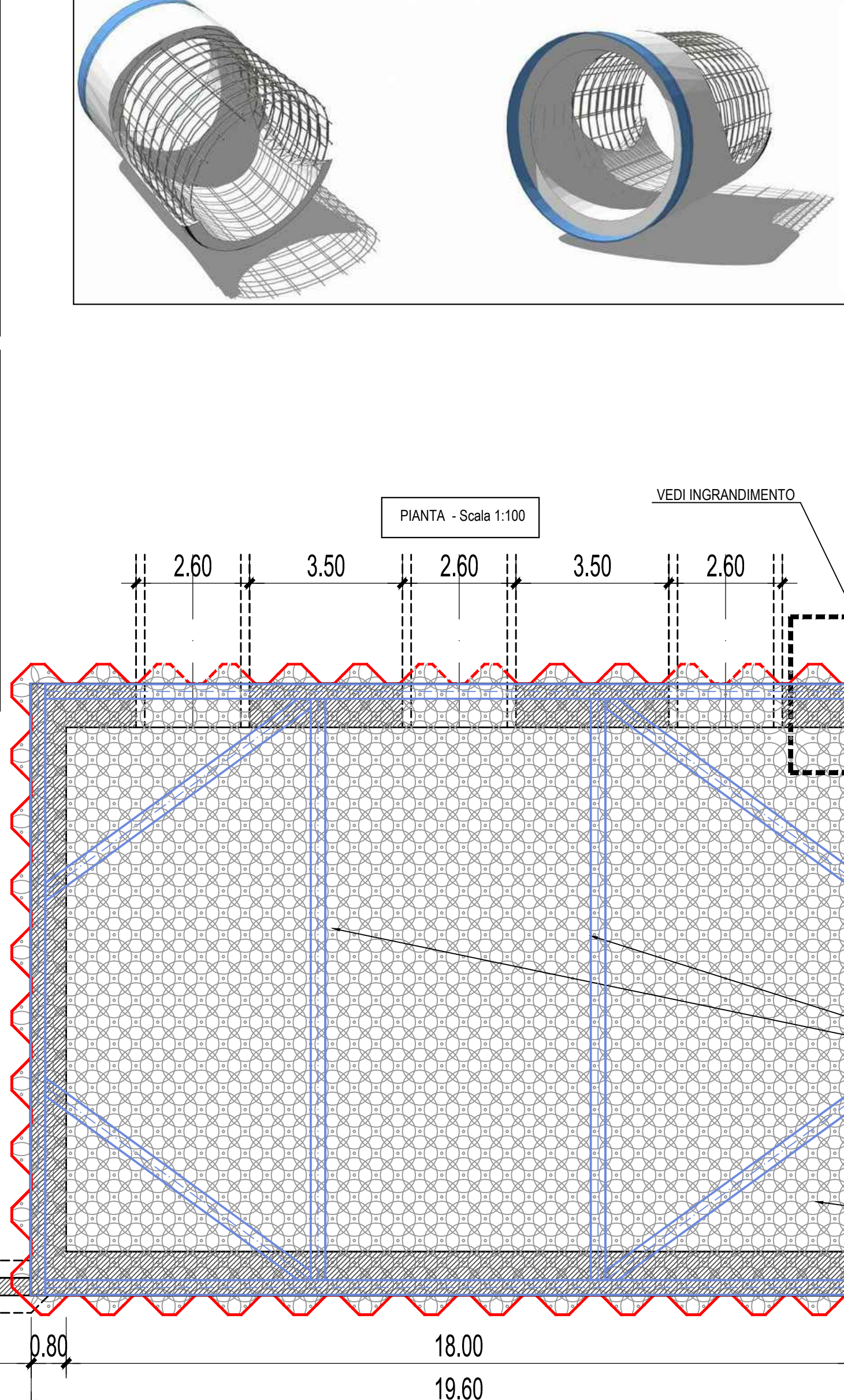
Rivestimento interno in liner polietilenico ad alta densità (HDPE)
